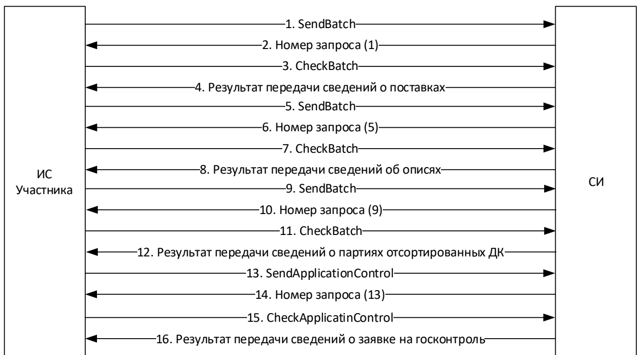
Рисунок 17 – Схема процесса взаимодействия с СИ при сортировке ДК
