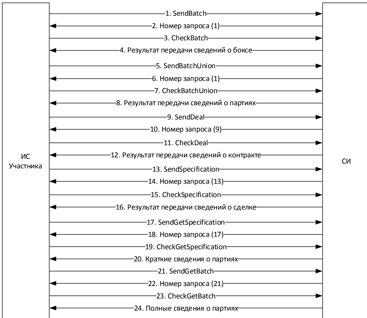
Рисунок 17 – Схема процесса взаимодействия с СИ
