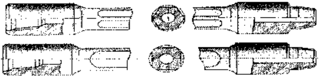
Рис. 133.2. Внешний вид ведущих бурильных труб
