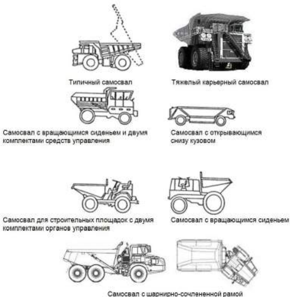
Рис. 189.1. Примеры самосвалов
