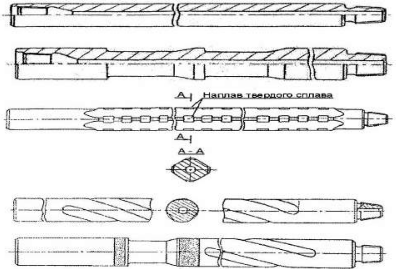
Рис. 133.1. Внешний вид утяжеленных бурильных труб
