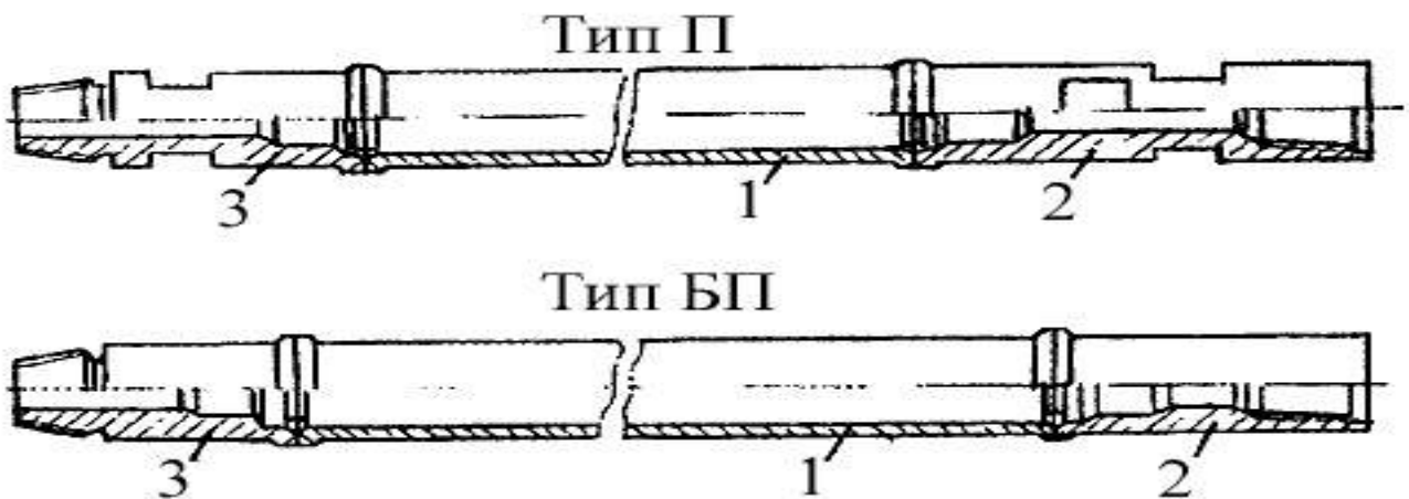
Рис. 133.3. Внешний вид бурильных труб
