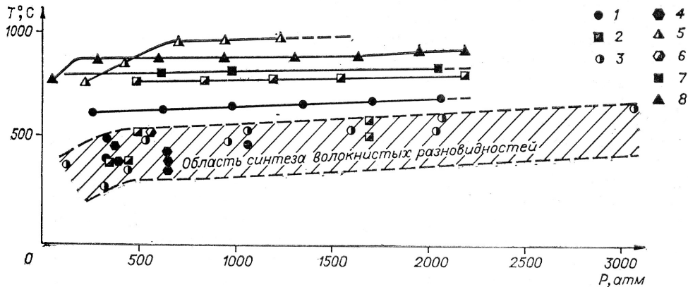
Рис. 53. P — T диаграмма синтетических волокнистых и микропризматических амфиболов (по Д. В. Калинину, 1971).
