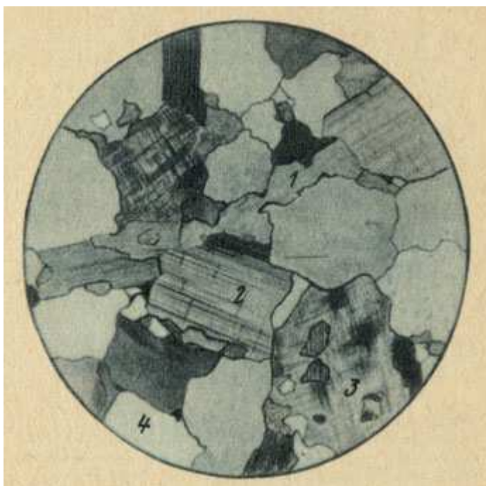
Рис. 14. Шлиф гранита под микроскопом. 1 - слюда, 2 - калиевый шпат, 3 - плагиоклаз, 4 - кварц
