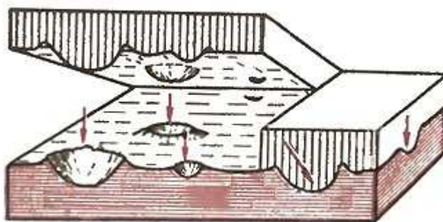
Рис. 28. Слой глинистого сланца с ямками от дождевых капель и
