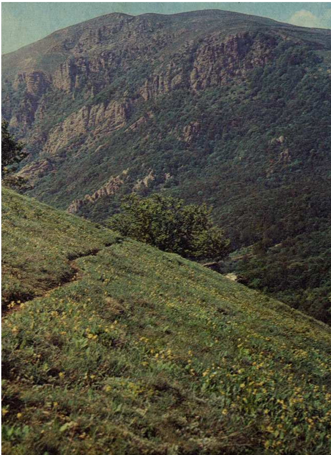
Рис. 12. Скалистые обрывы известняков Главной гряды Крымских гор (на дальнем плане), урочище Джурла
