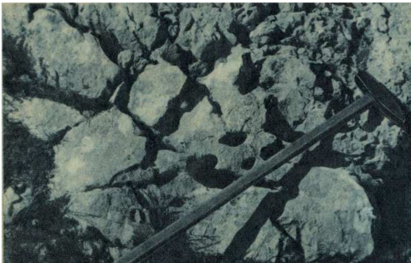
Рис. 8. Известняк с пустотами, следами растворения водой. Гора Чатыр-Даг, Крым
