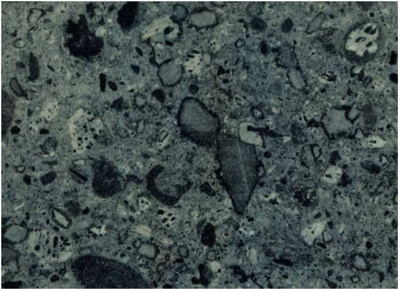
Рис. 21. Полированная поверхность образца якутского кимберлита с хорошо видимым обломочным строением
