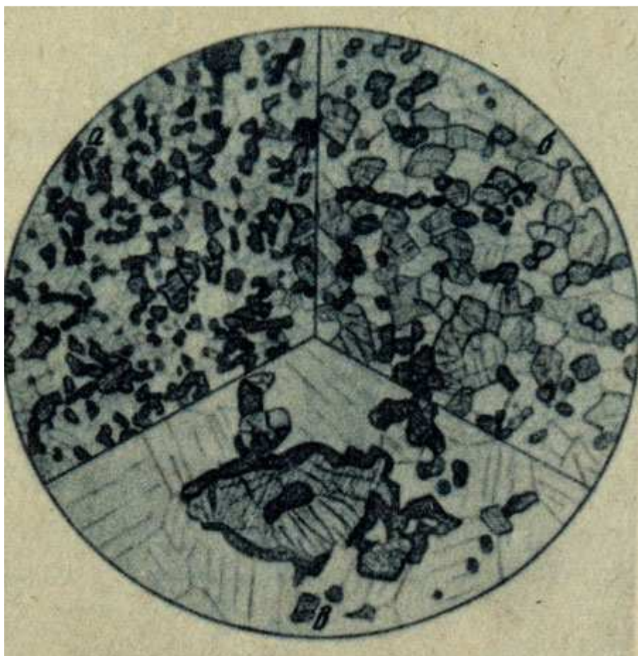
Рис. 22. Гранат - пироксен - плагиоклазовый роговик под микроскопом. По Ю. И. Половинкиной и др. а - тонкозернистый роговик, б - мелкозернистый роговик, в - среднезернистый роговик
