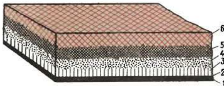
Рис. 41. Схема разрушения облицовки из натурального камня. 1 - внешняя корка, 2 - первоначальная поверхность камня, 3 - внутренняя корка, 4 - пылевато-мучнистый разрушенный слой, 5 - переходная зона, 6 - неповрежденный камень
