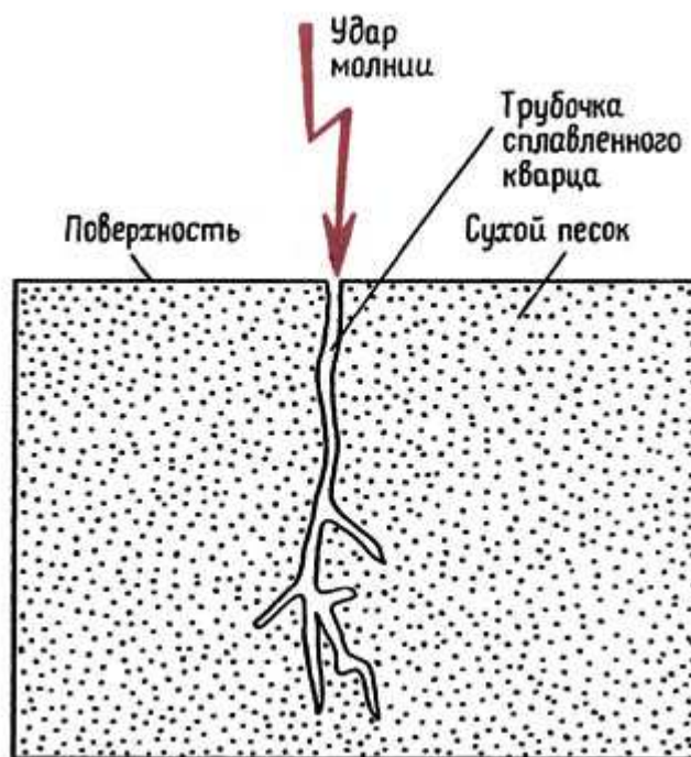
Рис. 27. Схема образования фульгурита
