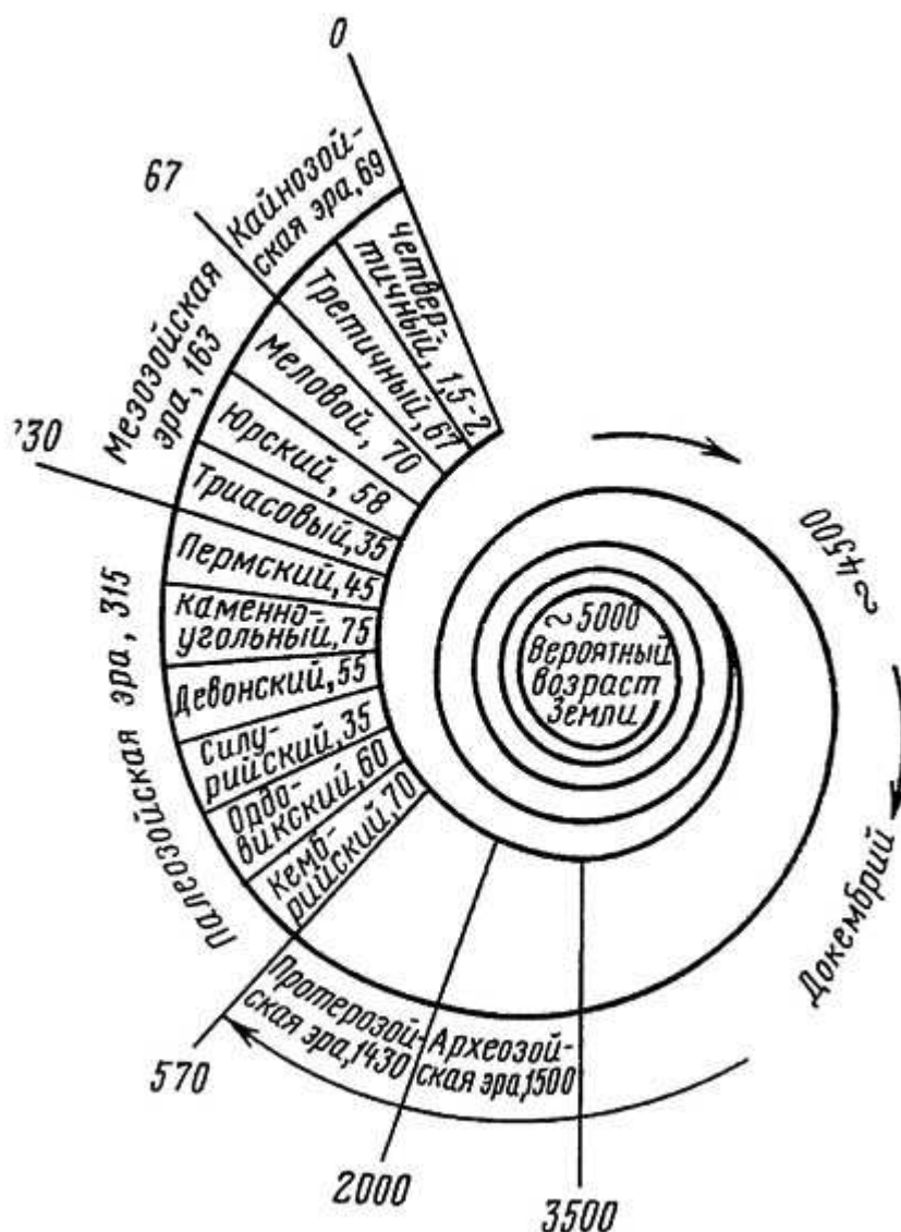
Рис. 2. Абсолютный возраст Земли и геологических периодов в миллионах лет. По К. И. и В. К. Лукашовым, с изменениями
