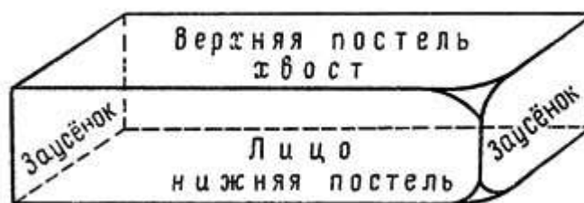
Рис. 25. Заготовка монолита гранита и ее части
