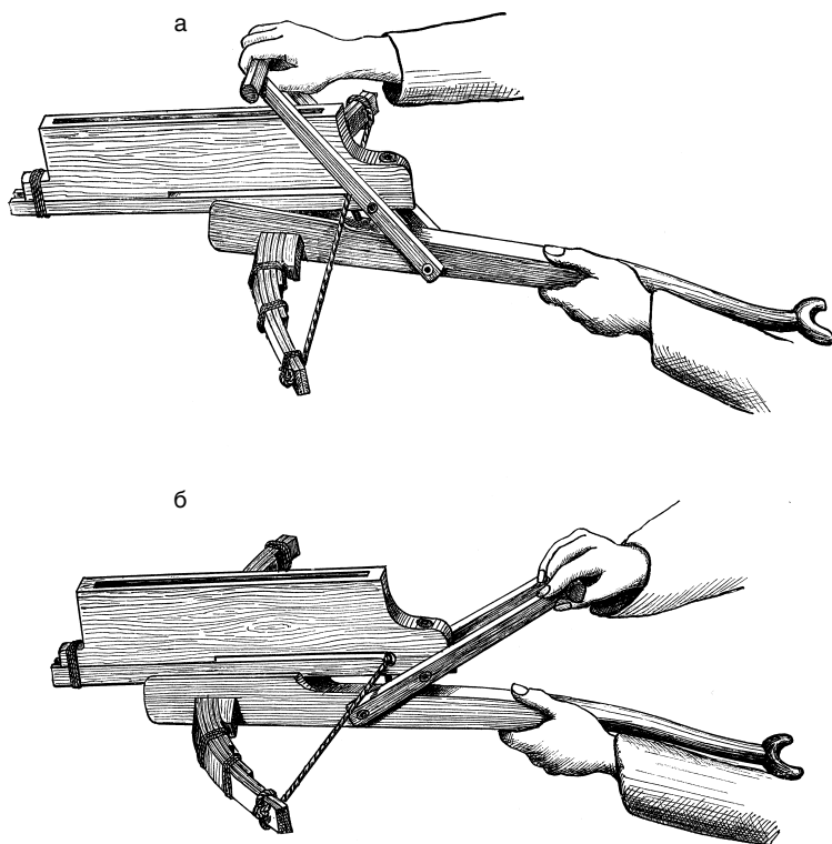
Рис. 87. Действие китайского арбалета: а — магазин, полный стрел, проталкивается рычагом вперед. Тетива удерживается в пазе над спусковым механизмом; б — арбалет в готовности к выстрелу. После нажатия нижнего выступающего конца спускового механизма по направлению к поверхности ложа тетива выталкивается из паза
